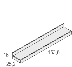
GALERÍA 154x16 cm
